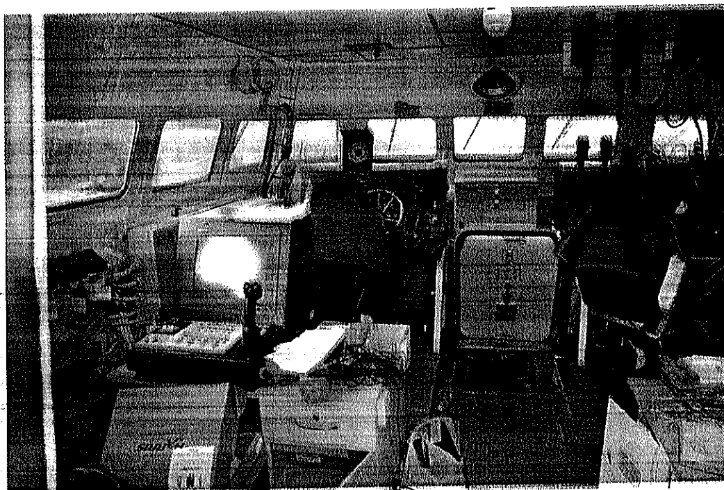
Фото № 3. Обзорный вид командной рубки малого бронированного артиллерийского катера «Никополь».
