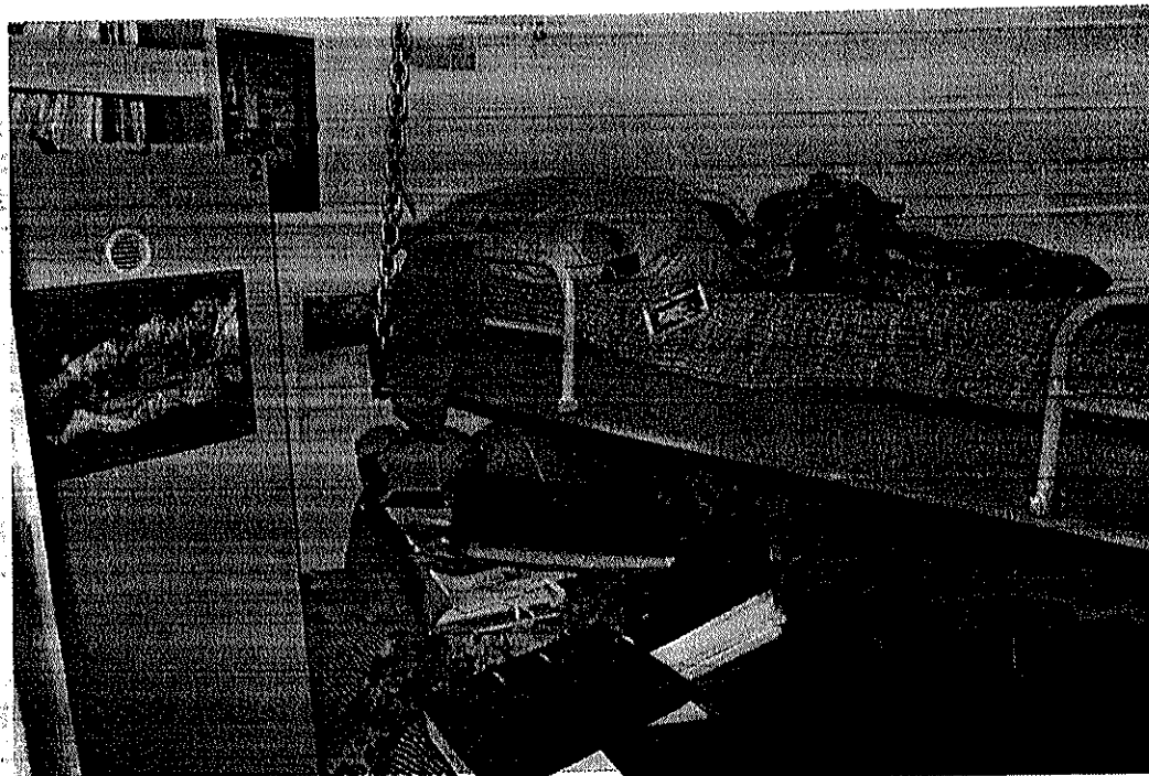
Фото № 4. Обзорный вид каюты малого бронированного артиллерийского катера «Никополь».
