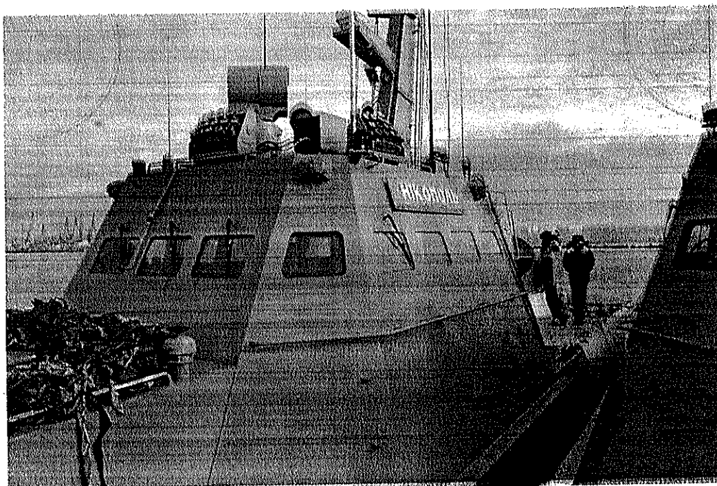
Фото № 2. Вид левого борта малого бронированного артиллерийского катера «Никополь».
