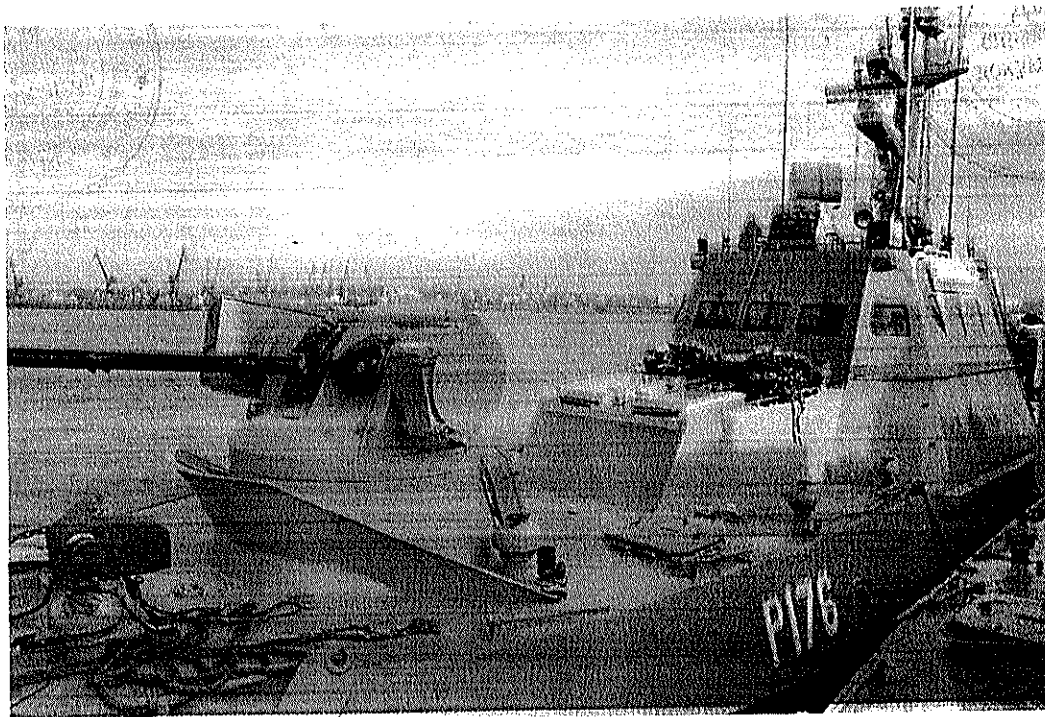
Фото № 1. Обзорный вид малого бронированного артиллерийского катера «Никополь».
